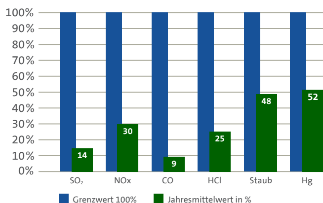
Jahresmittelwerte 2025 der kontinuierlich ermittelten Emissionen im Verhältnis zu den Grenzwerten der 17. BImSchV
