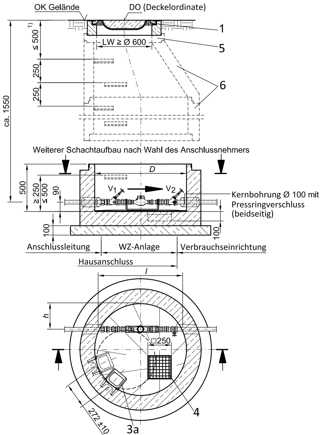
Bild 3 – Wasserzählerschacht aus Betonfertigteilen (Prinzipskizze)
