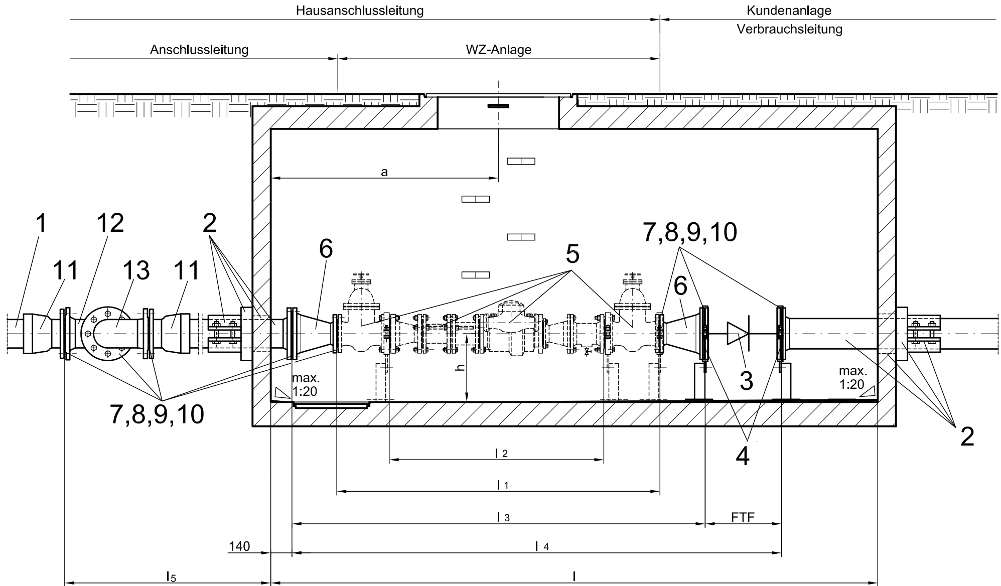
Bild 1 – Einbau einer Parallel-WZ-Anlage bei getrennter Verbrauchsleitung DN 80 – DN 300 (Bsp. Einbau Parallel-Verbund-WZ-Anlage DN 100 nach WN 289 in Anschlussleitung DN 200) (Prinzipskizze)
