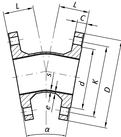
Bild 1 – Doppelflansch-Bögen (FFK) in Anlehnung an DIN EN 545 (Prinzipskizze, Bsp. FFK 30)
