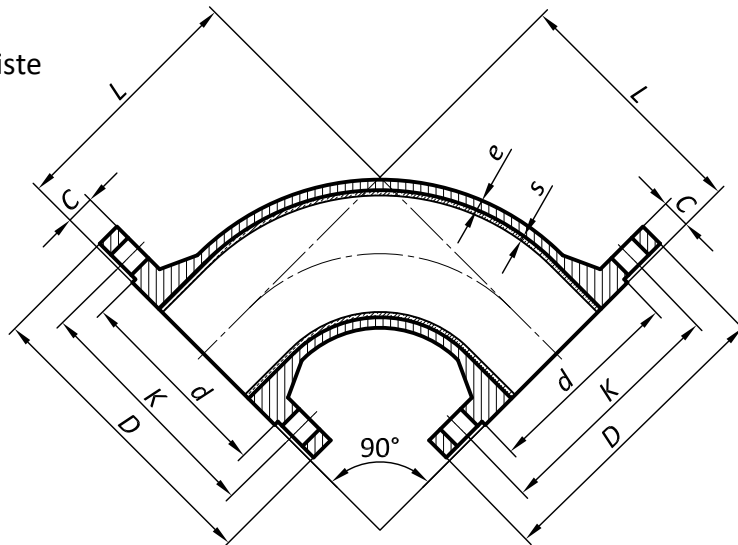
Bild 1 – Doppelflansch-Bogen 90° (Q) nach DIN EN 545 (Prinzipskizze)
