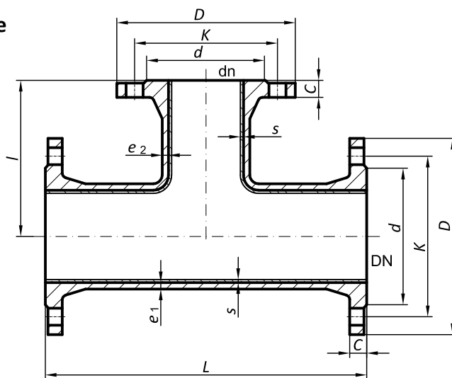
Bild 1 – Flansch-T-Stück DIN EN 545 (Prinzipskizze)
