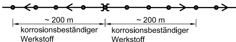
R-Kanal (Variante: mehrere Haltungen nach einem hydraulischen Hochpunkt)
