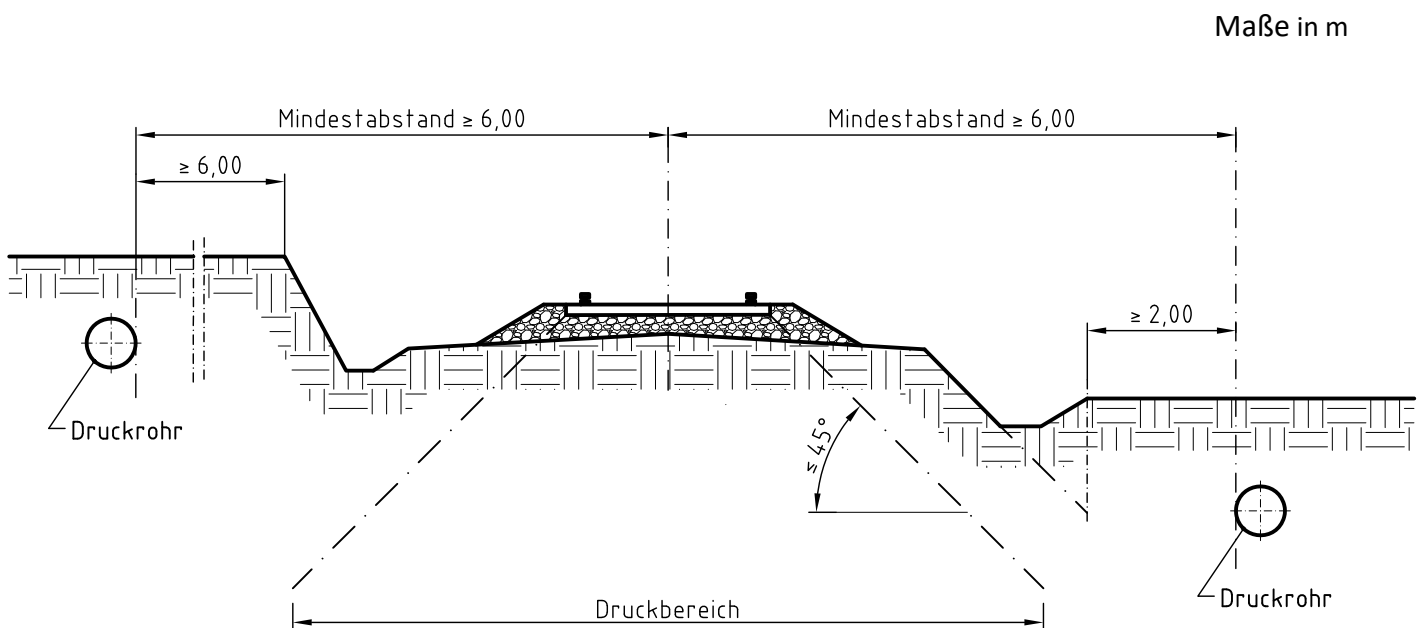
Bild 3 – Mindestabstände bei Leitungslängsführungen (Richtlinien 2012:2017-07, 877.2201 in Anlehnung an Bild 2) (Prinzipskizze)
