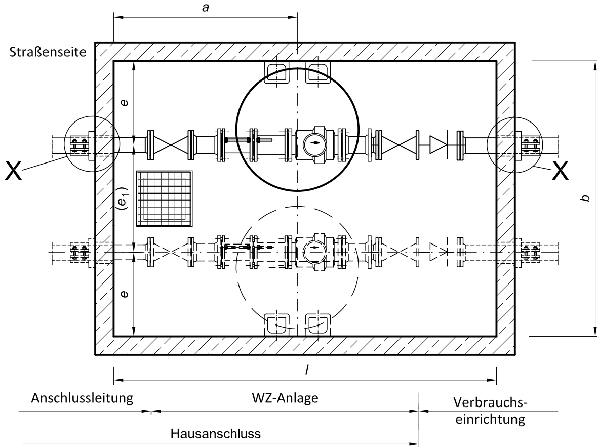
Bild 1 a – Draufsicht für Wasserzählerschacht; Beispiel für Einbau einer Groß- bzw. Parallel-Groß-WZ-Anlage DN 200, DN 300 bzw. DN 400 nach Bild 1 (Prinzipskizze für einen Hausanschluss)
