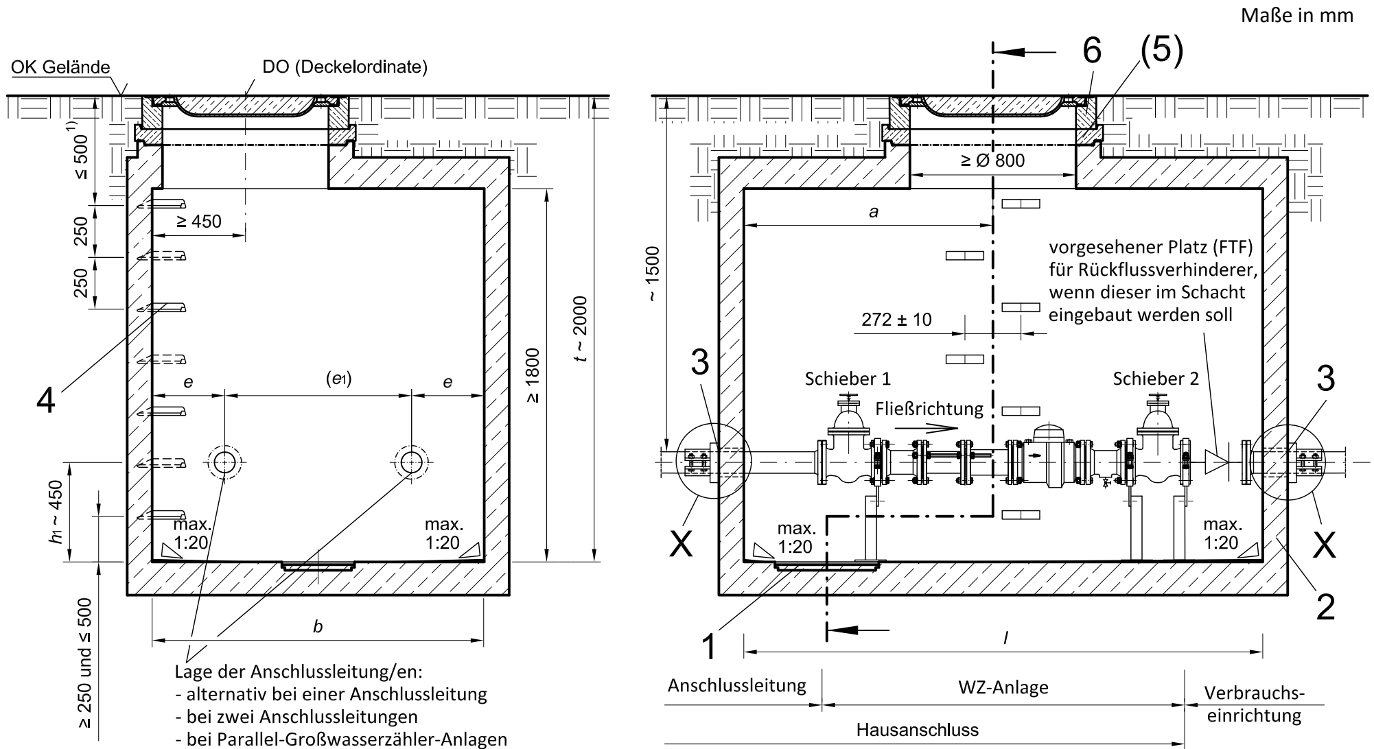
Bild 1 – Wasserzählerschacht – Beispiel für Einbau einer Groß- bzw. Parallel-Groß-WZ-Anlage DN 200, DN 300 bzw. DN 400 (Prinzipskizze)
