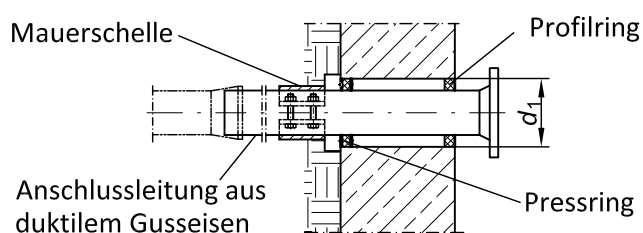
Bild 2 – Detail X: Wanddurchführungen am Wasserzählerschacht (Prinzipskizze)
