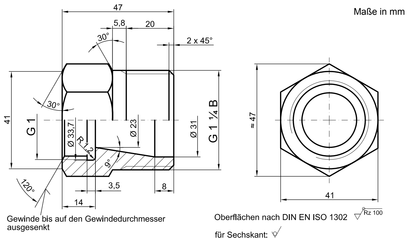
Bild 1 – Kleines Übergangsstück G 1 ¼ B x G 1 (Prinzipskizze)
