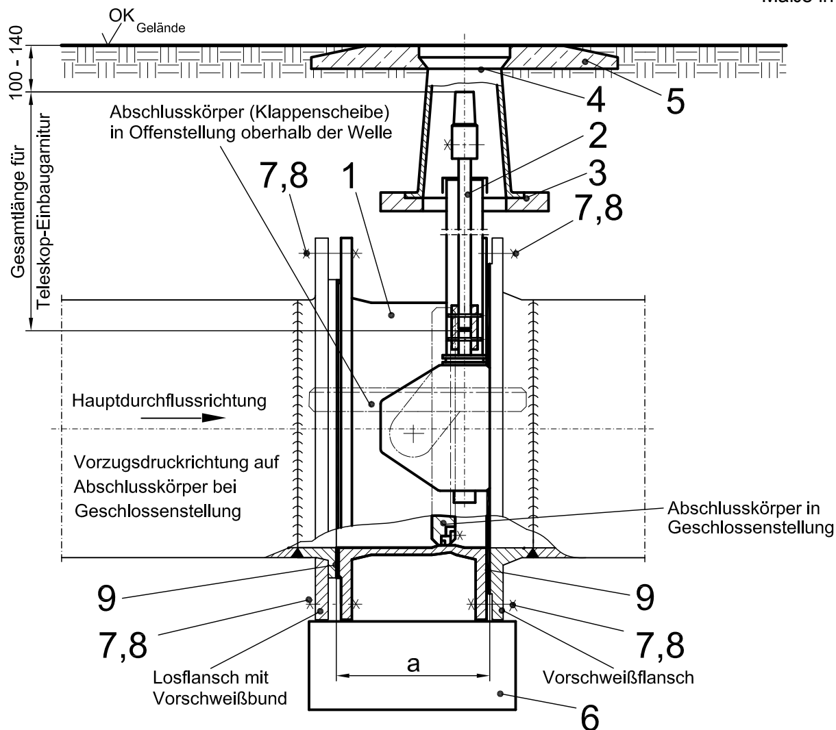
Bild 1 – Einbaudarstellung einer Klappe (Prinzipskizze)
