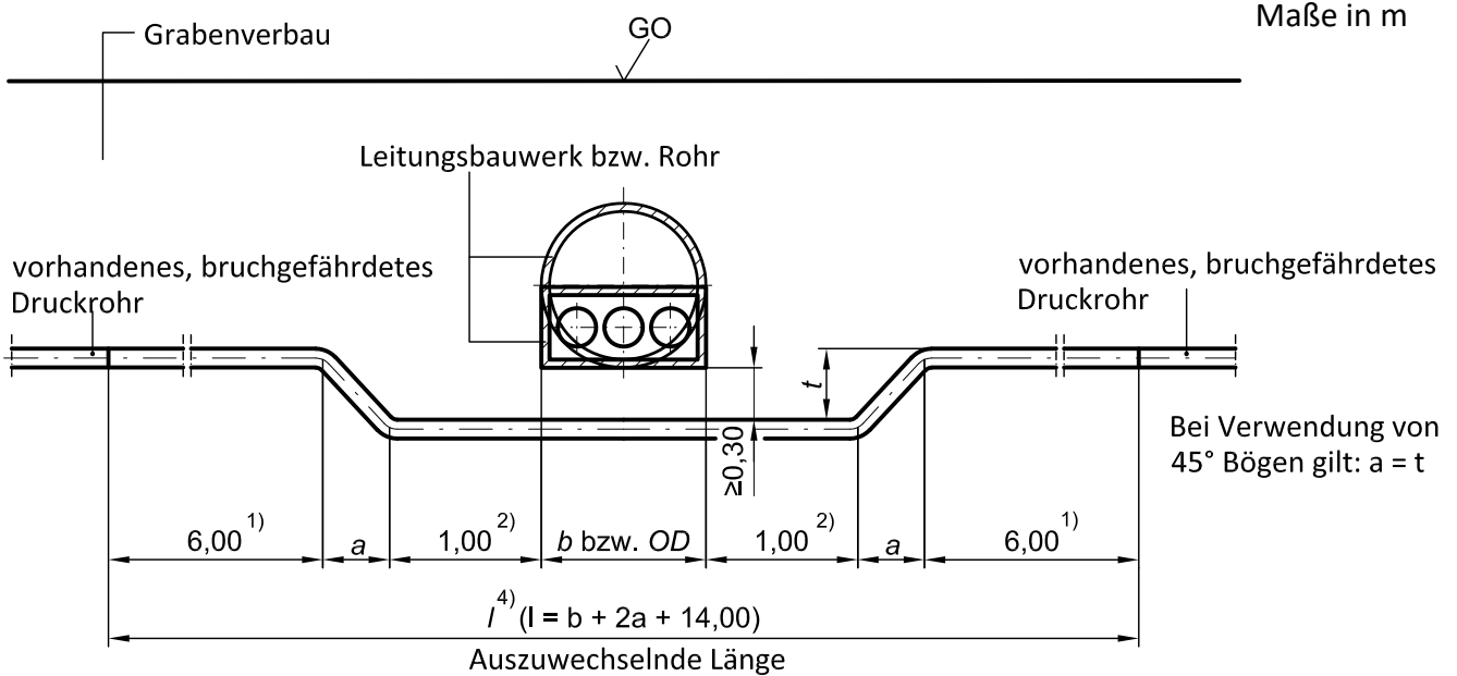
Bild 5 – Neu zu errichtendes Leitungsbauwerk bzw. Rohr gleich bzw. höher liegend als vorhandene bruchgefährdete Druckleitung (Prinzipskizze)
