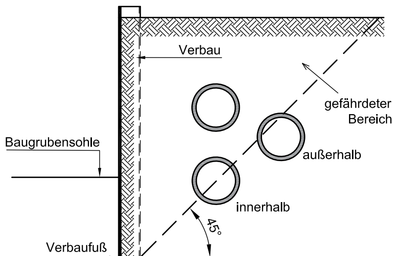
Bild 1 – Grenzbereich der Lage einer bruchgefährdeten Leitung in Bezug auf den gefährdeten Bereich (Prinzipiskizze)
