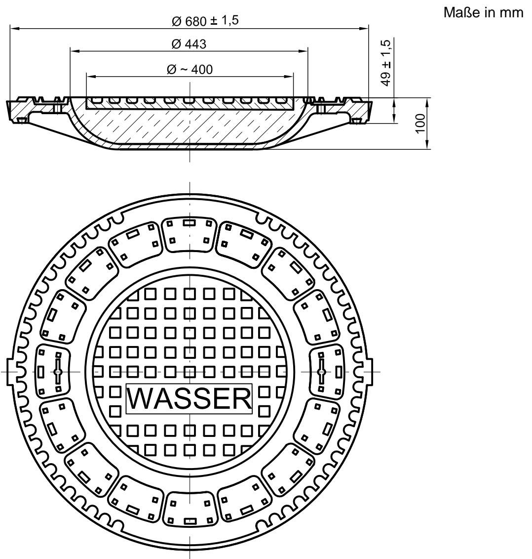
Bild 1 – Deckel ähnlich DIN 19584-2, ohne Lüftungsöffnungen, mit Einlage DIN 19584-4, mit Beschriftung 1)
